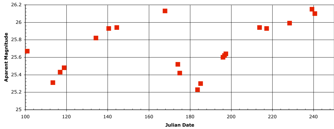
Galaxy 4, Cepheid 3
