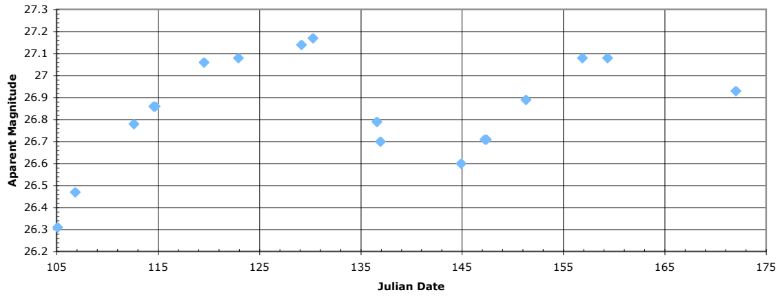
Galaxy 4, Cepheid 2
