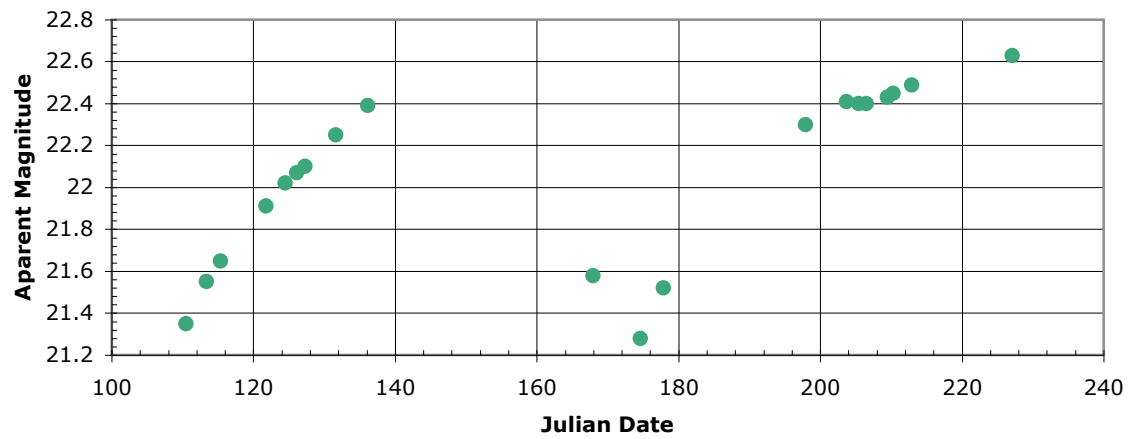
Galaxy 2, Cepheid 3
