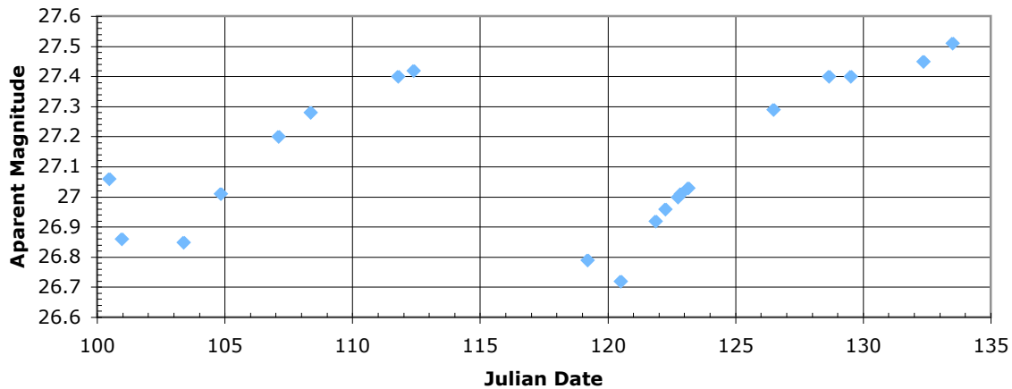
Galaxy 3, Cepheid 2
