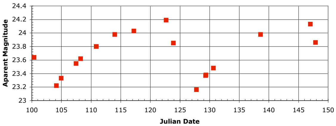
Galaxy 2, Cepheid 3
