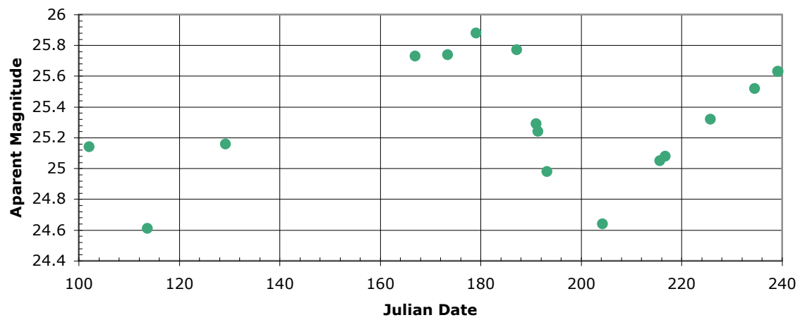
Galaxy 4, Cepheid 3
