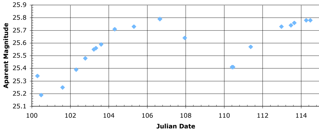
Galaxy 2, Cepheid 2
