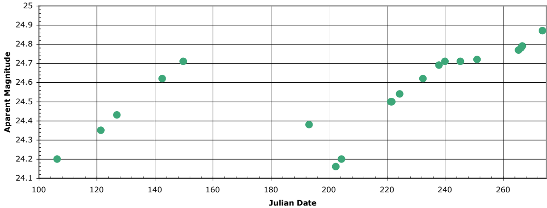
Galaxy 3, Cepheid 3
