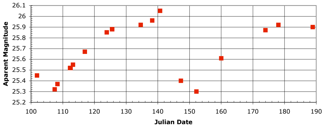
Galaxy 3, Cepheid 2
