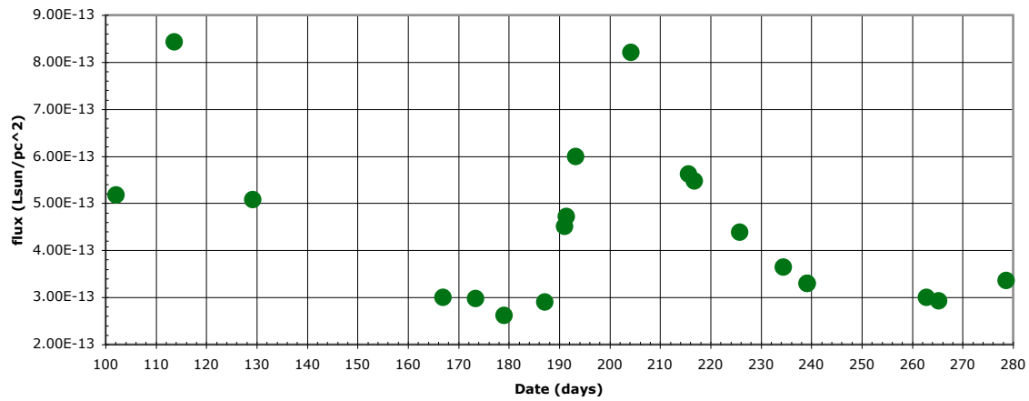
Galaxy 4 Cepheid 3
