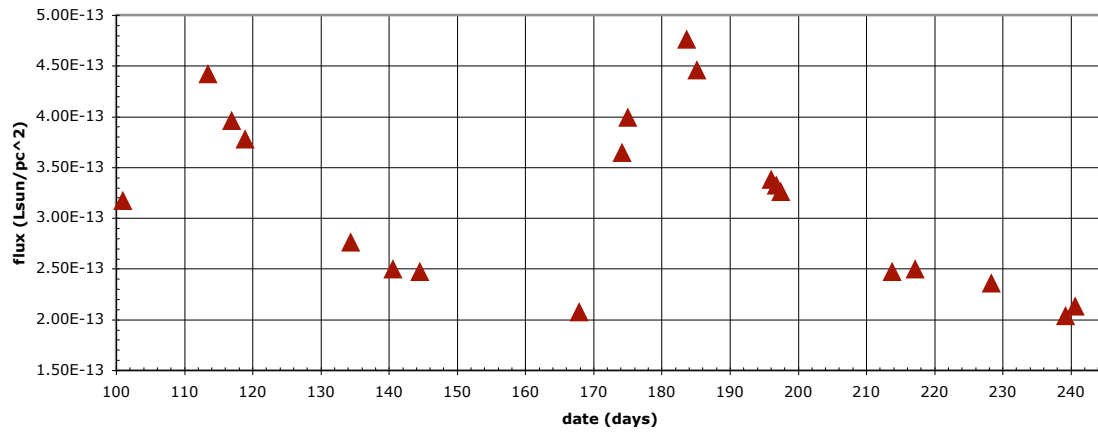
Galaxy 4 Cepheid 3
