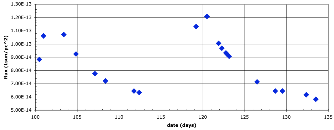
Galaxy 3 Cepheid 2
