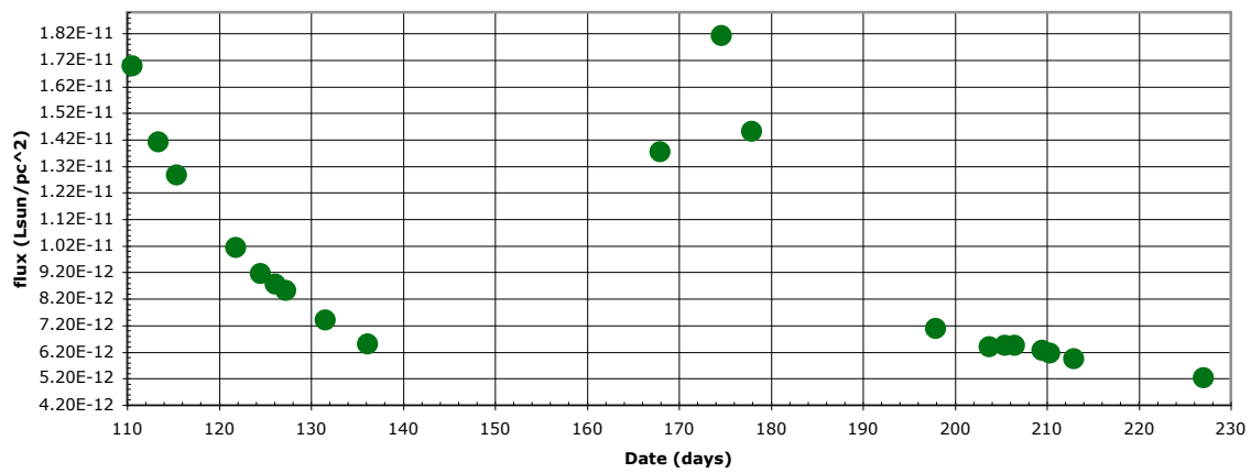
Galaxy 2 Cepheid 3
