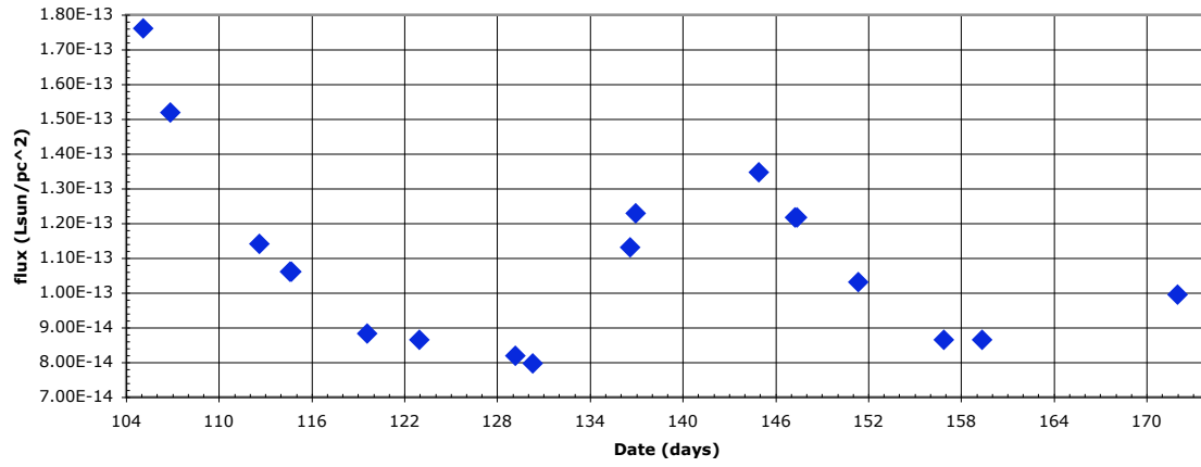
Galaxy 4 Cepheid 2
