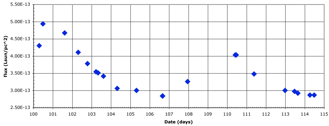
Galaxy 2 Cepheid 2
