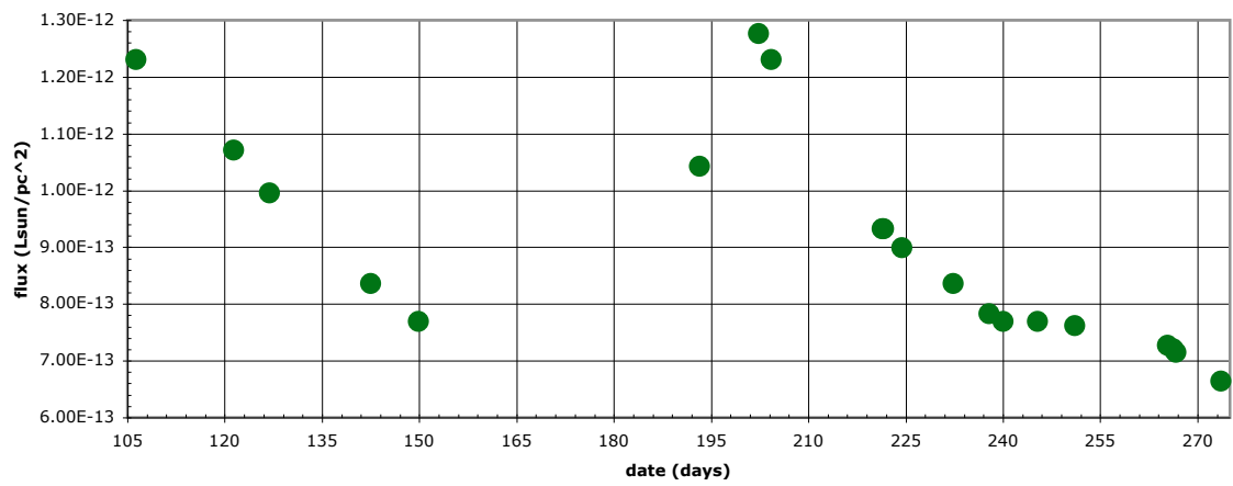
Galaxy 3 Cepheid 3
