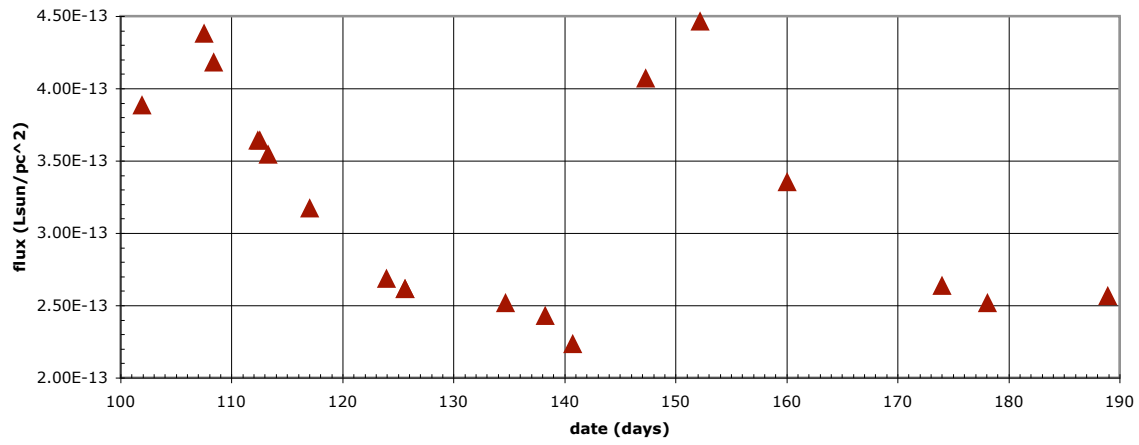
Galaxy 3 Cepheid 3
