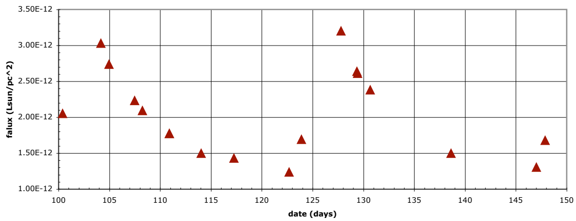
Galaxy 2 Cepheid 3
